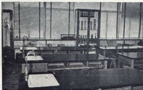
生物實驗室
