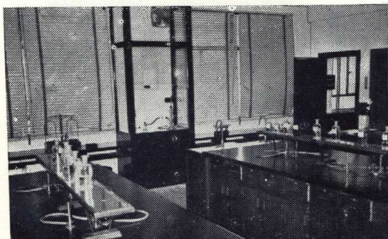
化學實驗室
